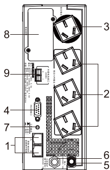
MT1000S 后面板(图三)
