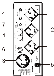
MT500 后面板(图二)
