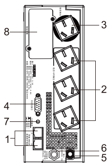
MT1000 后面板(图四)
