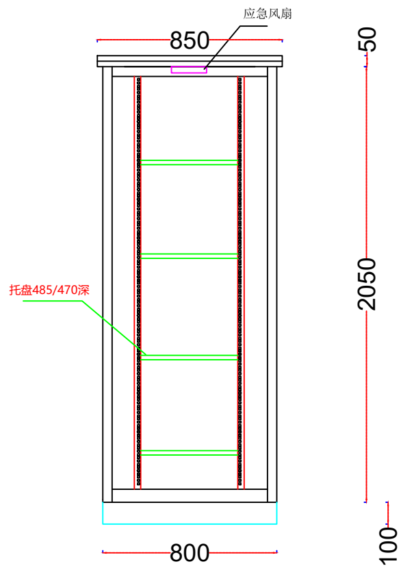
前视内部图
