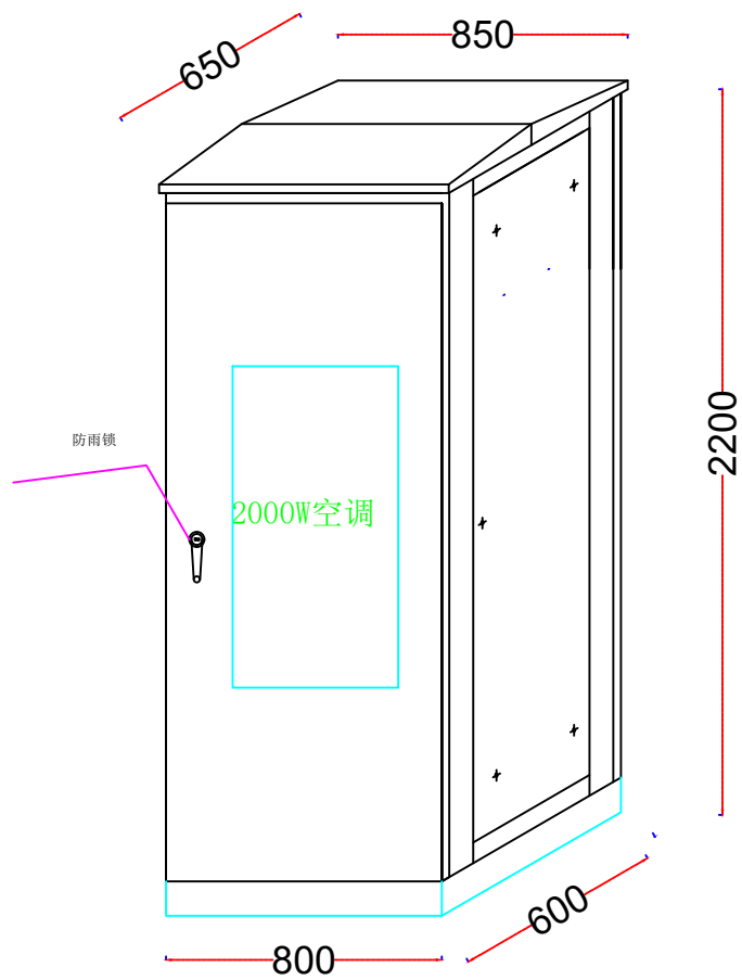
前视图
