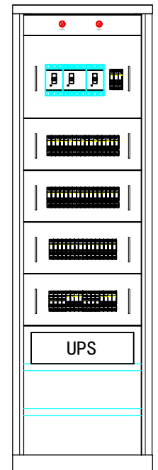
UPS电源一体柜 W600*H2000*D850
