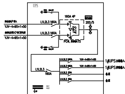
UPS输入配电柜系统图
