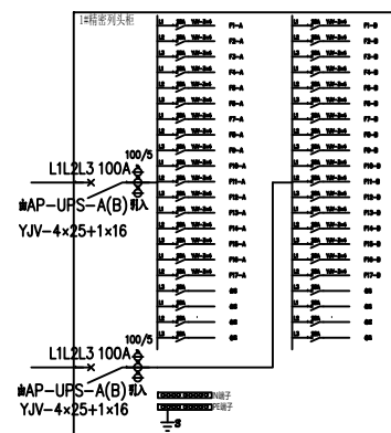
机房精密配电列头柜系统图
