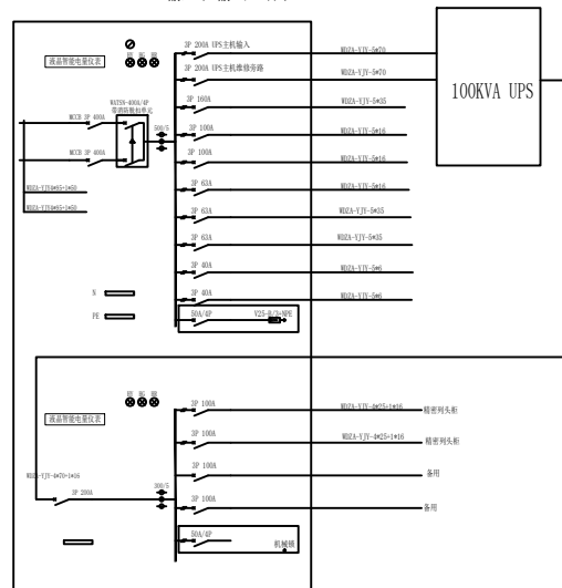
100KVA UPS输入和输出一体柜
