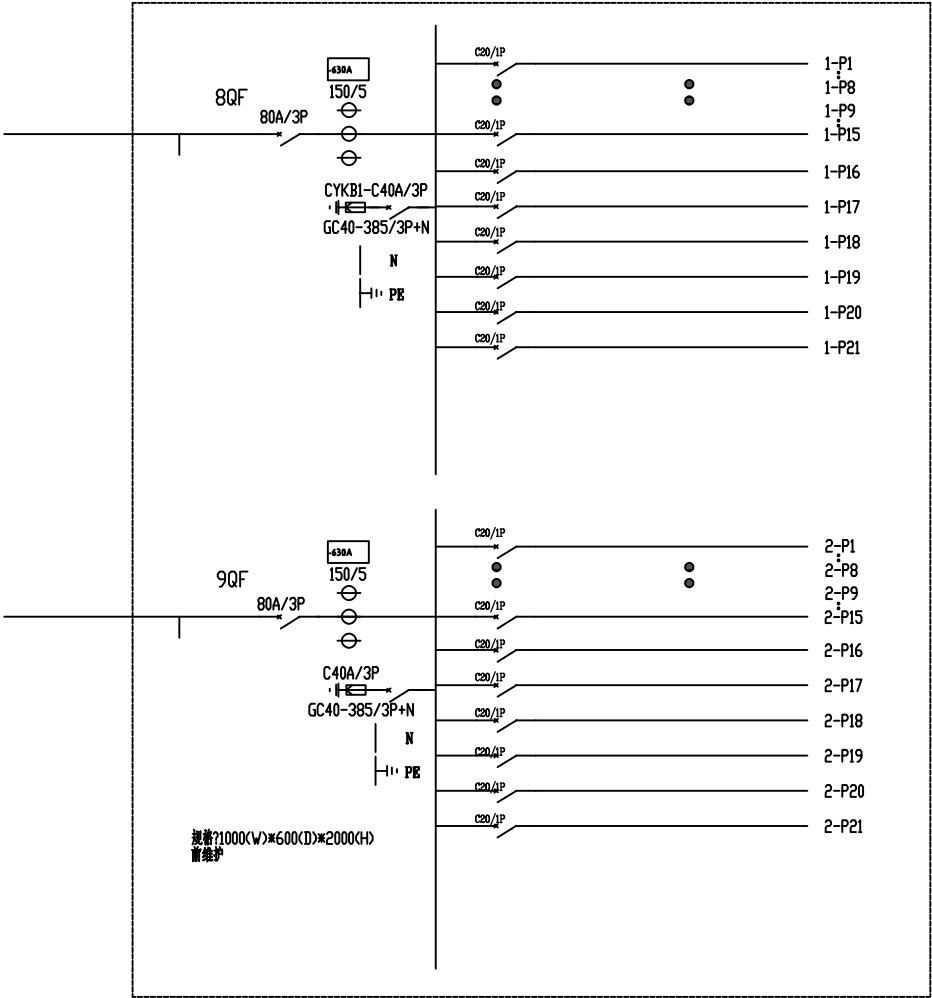
UPS列头配电柜系统图
