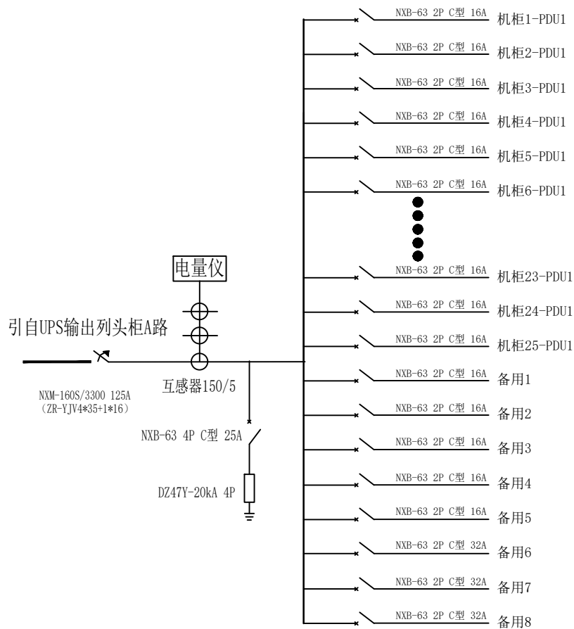
外接铜排部分示意
