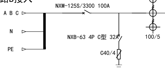
外接铜排部分示意
