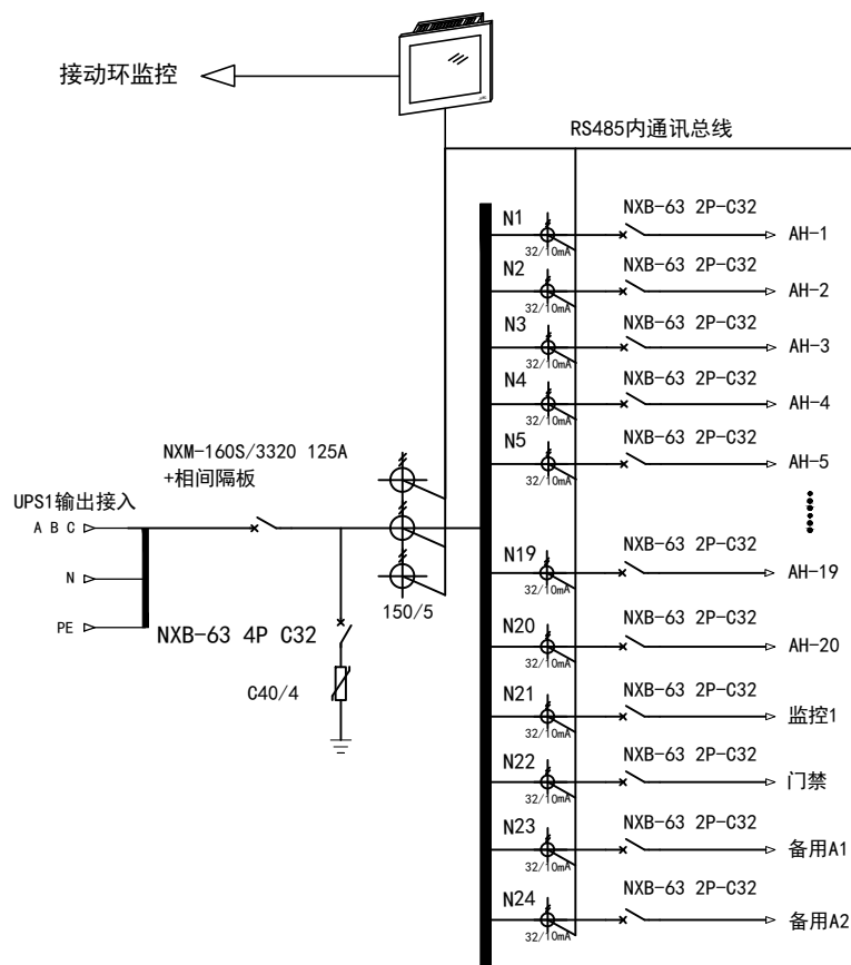
外接铜排部分示意
